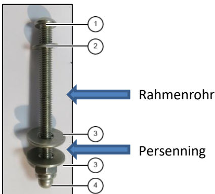
Abb. 1: Verschraubung
